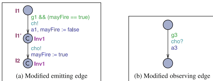
Fig. 13 Edge modifications for Fig. 12
